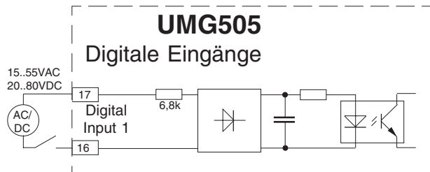
Abb.: Digital Input 1 für Gleich- und Wechselspannung .
