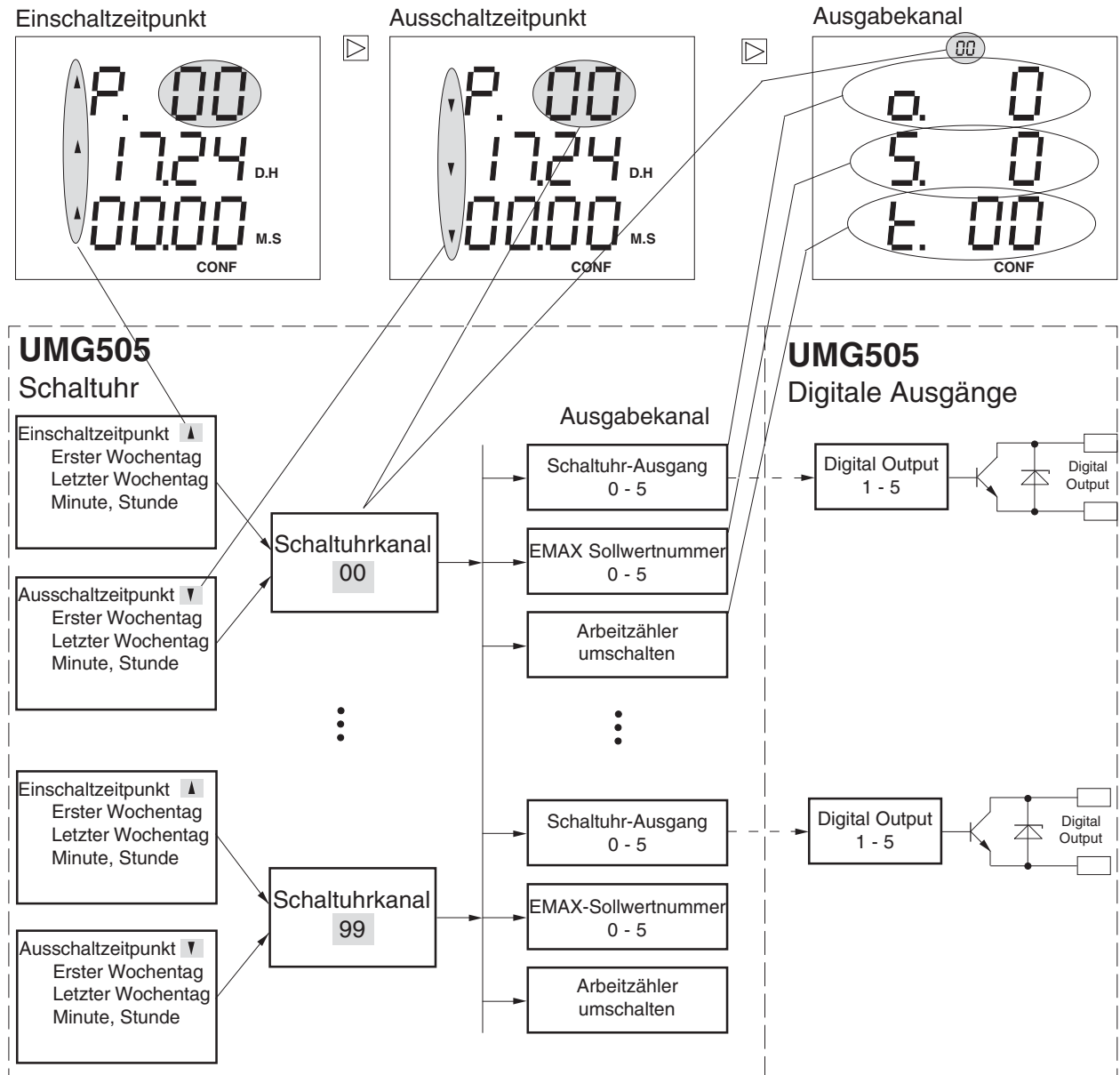
Abb. Blockschaltbild Schaltuhr
