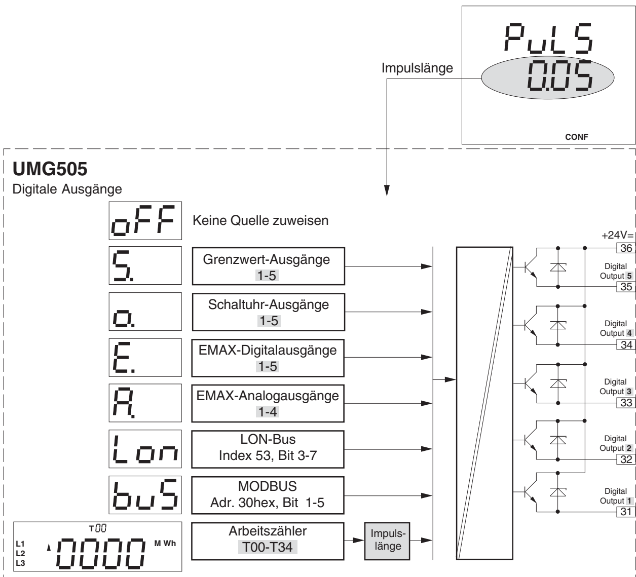
Abb. Blockschaltbild Digitale Ausgänge
