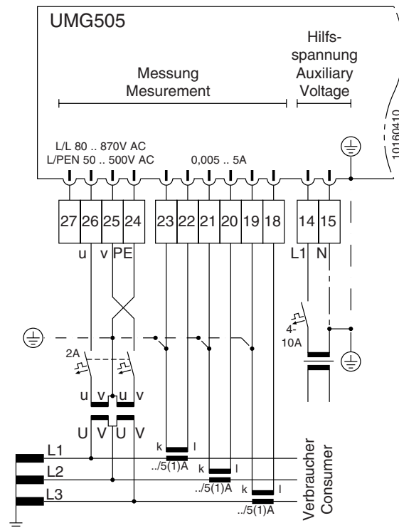
Abb. 2 Mittelspannungsseitige Messung mit zwei Spannungswandlern und drei Stromwandlern.
