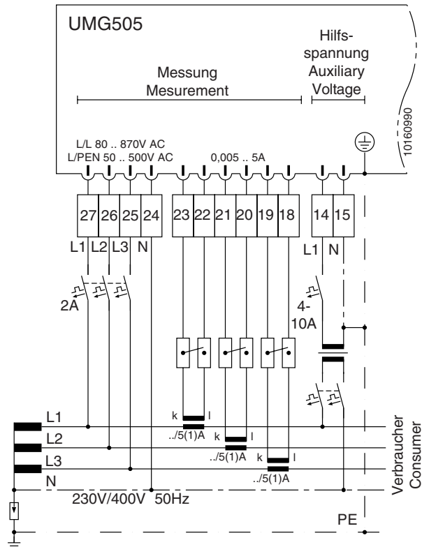
Abb. 5 Messung im IT-Netz mit N.
