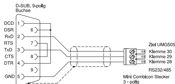
Abb. Anschlussbelegung RS232-Kabel (Option)
