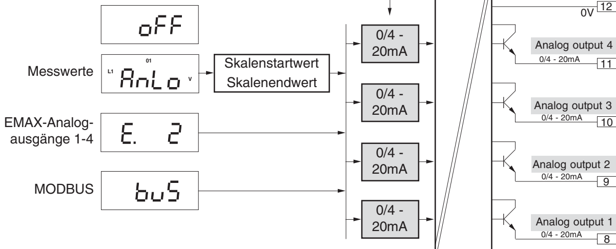
Abb. Blockschaltbild Analogausgang. Ausgabebereich einstellen.
