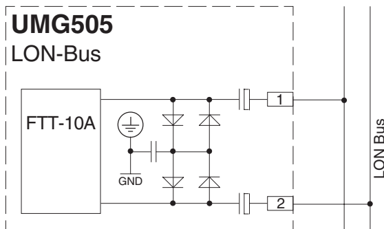
Abb. Anschlussbelegung LON-Bus
