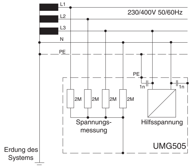
Abb. Prinzipialschaltbild UMG505 im TN-Netz.
