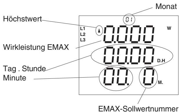
Abb.: Mittelwertbildung für die Wirkleistung EMAX über eine Messperiode von 15 Minuten.
