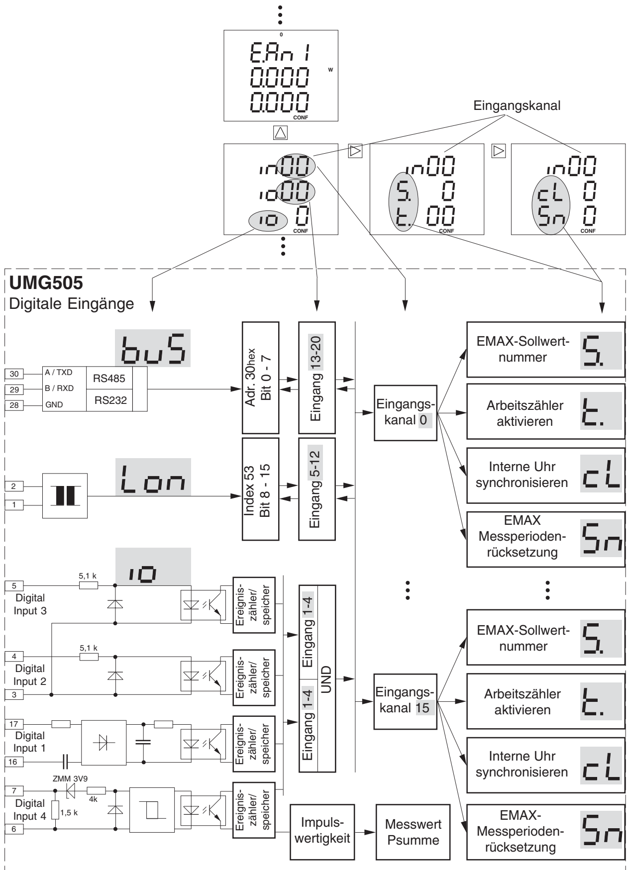
Abb. Blockschaltbild Digitale Eingänge
