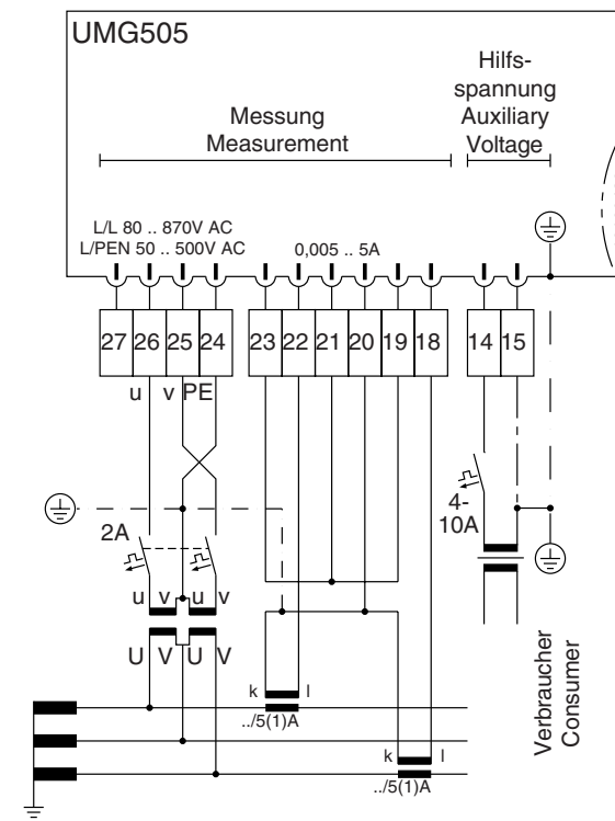
Abb. 4 Mittelspannungsseitige Messung mit zwei Spannungswandlern und zwei Stromwandlern.
