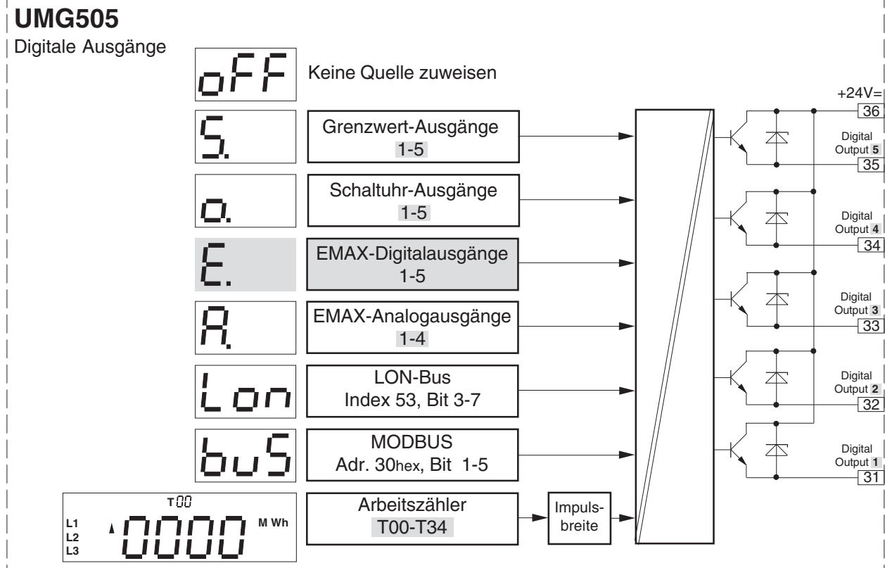
Abb. Blockschaltbild Digitale Ausgänge
