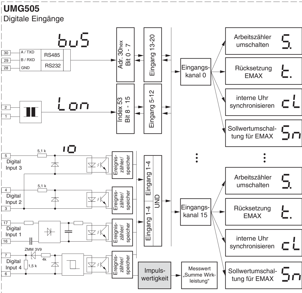
Abb. Blockschaltbild Digitale Eingänge
