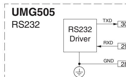
Abb. Anschlussbelegung RS232
