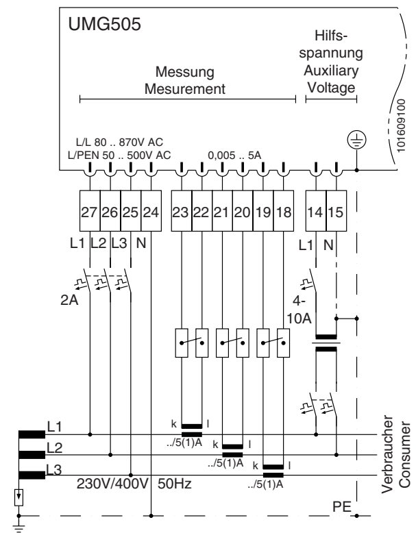
Abb. 6 Messung im IT-Netz ohne N.
