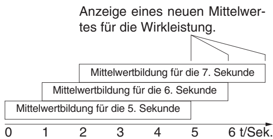
Abb.: Mittelwertbildung für die Wirkleistung über 5 Sekunden.
