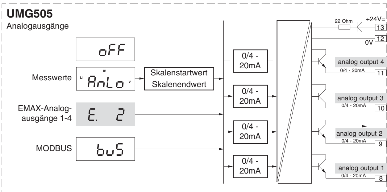
Abb. Blockschaltbild Analogausgang. Auswahl der Quelle.
