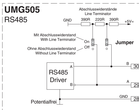
Abb.: Anschlussbelegung RS485
