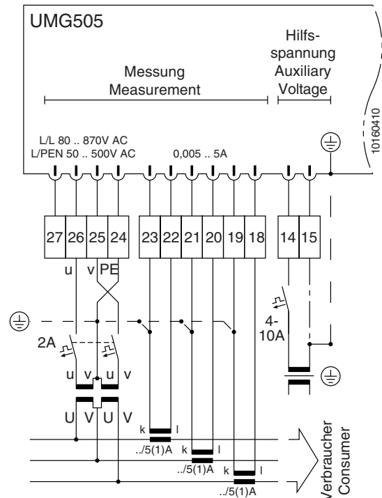
Abb. Aronschaltung mit zwei Spannungswandlern und drei Stromwandlern.
