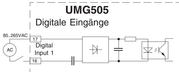
Abb.: Digital Input 1 nur für Wechselspannung .
