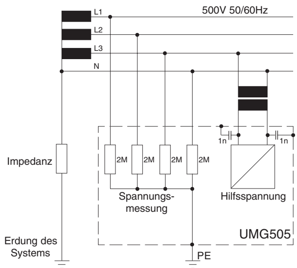
Abb. Prinzipialschaltbild UMG505 im IT-Netz mit N.
