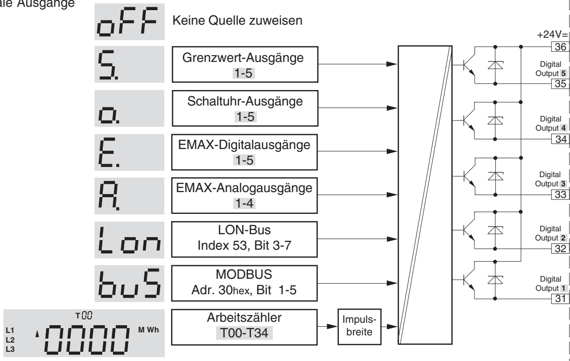
Abb. Blockschaltbild Digitale Ausgänge
