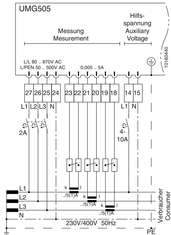
Abb. 7 Messung im TN-Netz über drei Stromwandler.
