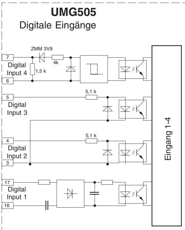
Abb.: Interne Schaltung der digitalen Eingänge.
