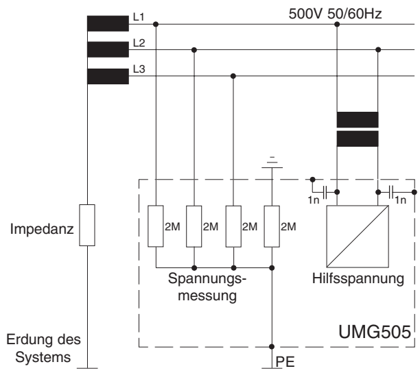
Abb. Prinzipialschaltbild UMG505 im IT-Netz ohne N.
