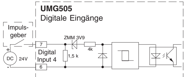
Abb.: Anschlussvorschlag; Digital Input 4 als Impuls-eingang.
