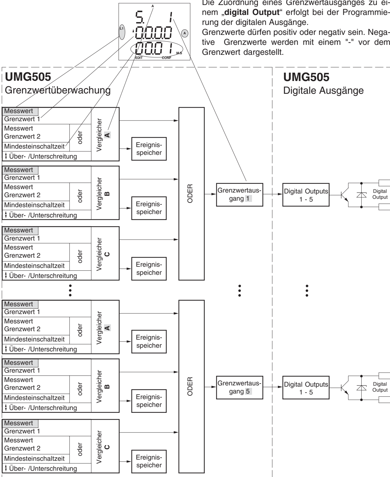
Abb. Bockschaltbild Grenzwertüberwachung.
