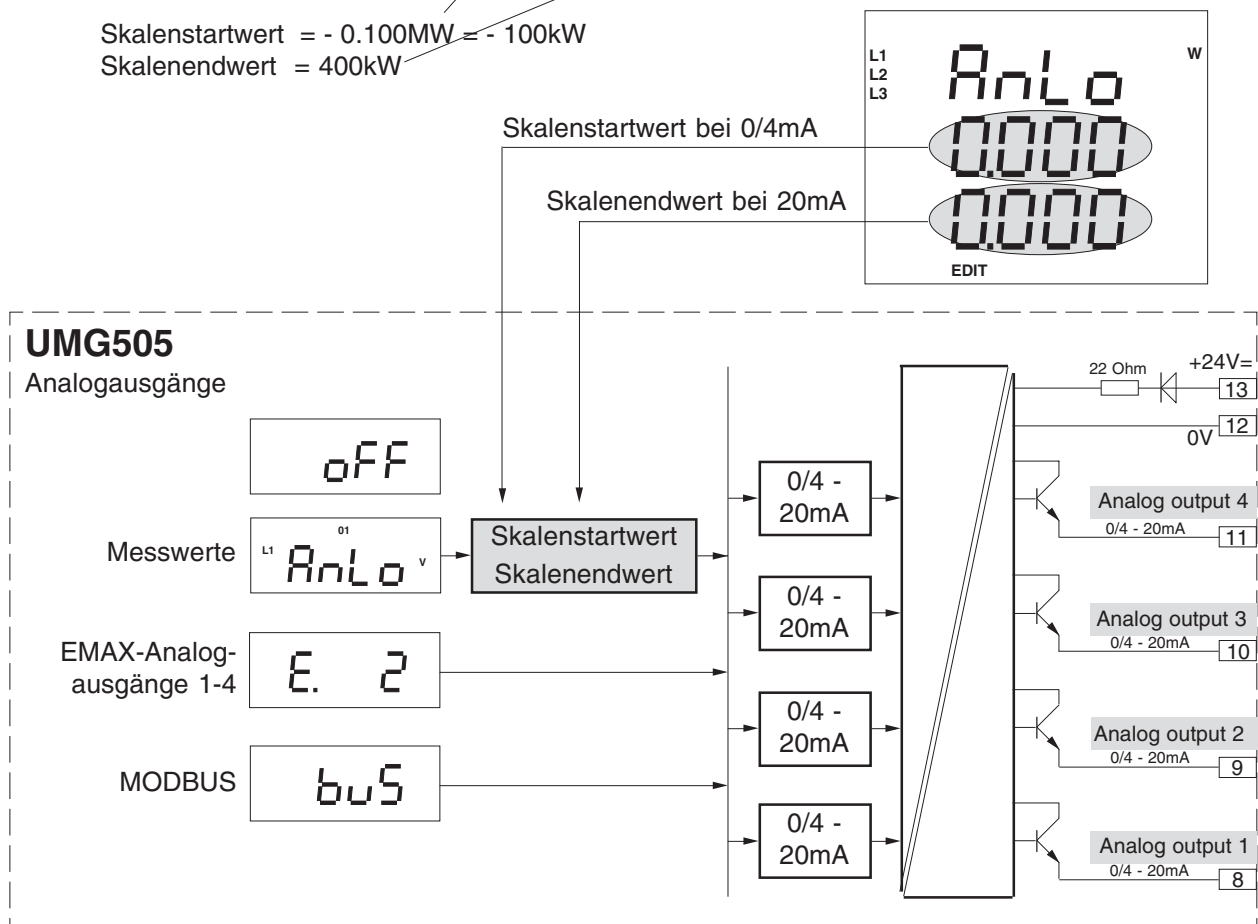
Abb. Blockschaltbild Analogausgang. Auswahl von Skalenstart- und Skalenendwert.
