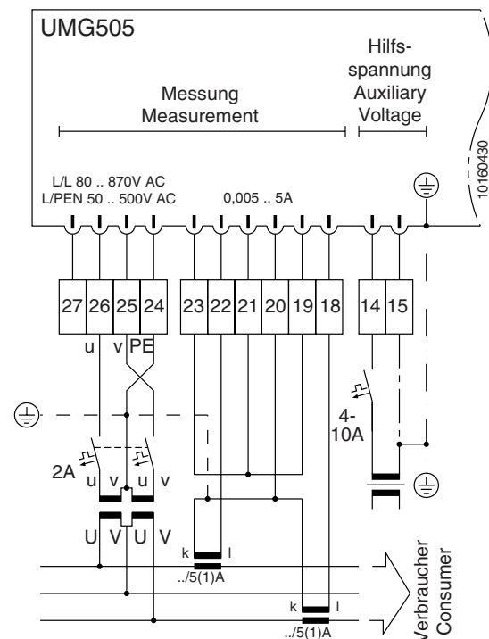
Abb. Aronschaltung mit zwei Spannungswandlern und zwei Stromwandlern.
