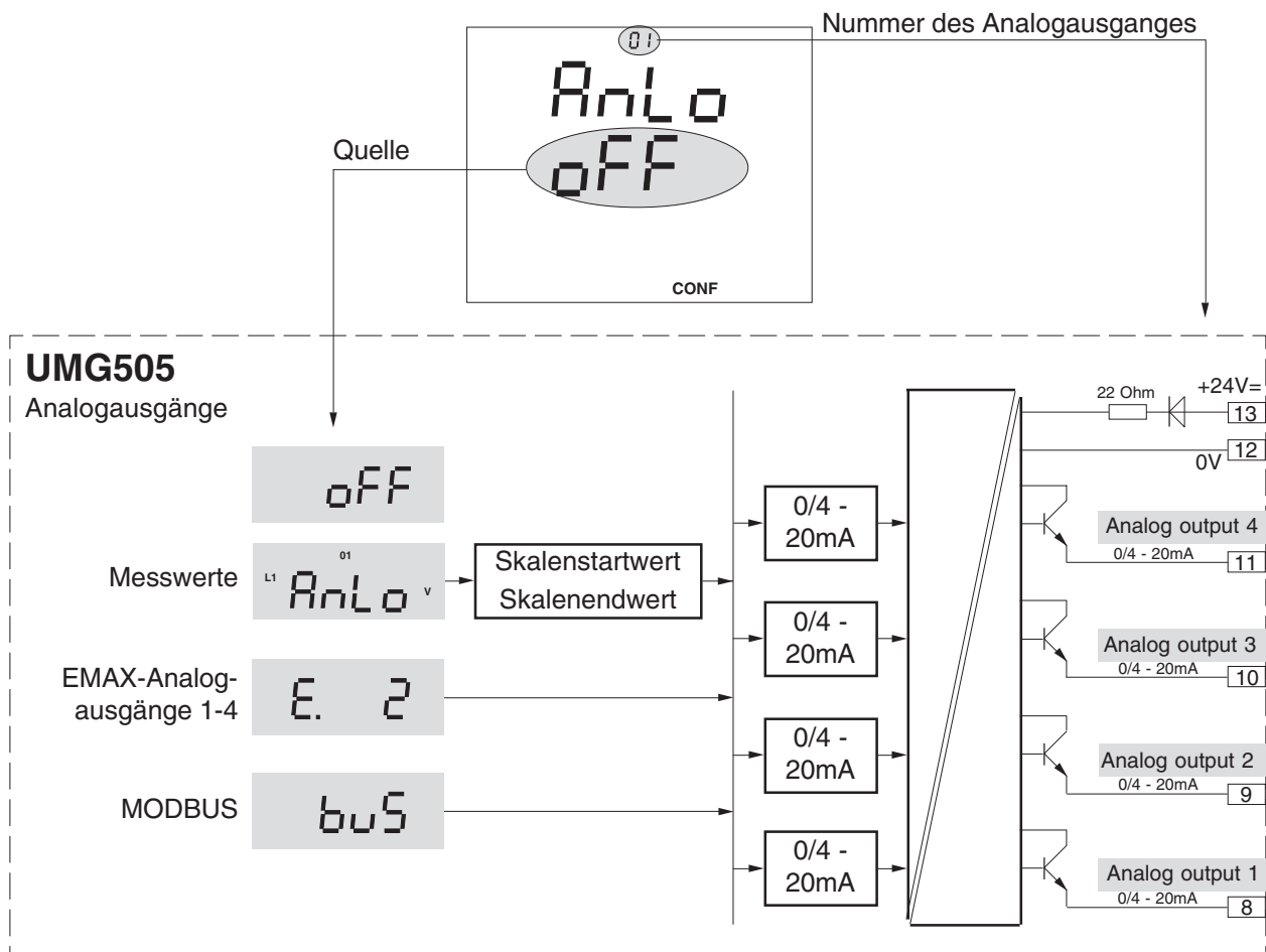
Abb. Blockschaltbild Analogausgang. Auswahl der Quelle.
