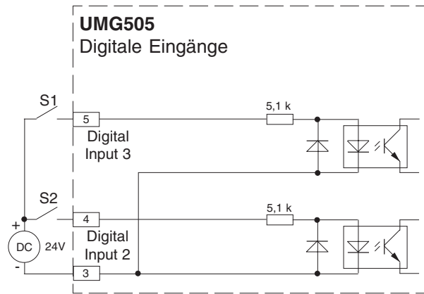
Abb.: Anschlussvorschlag; Digital Input 2 und 3 mit externer Hilfsspannung.
