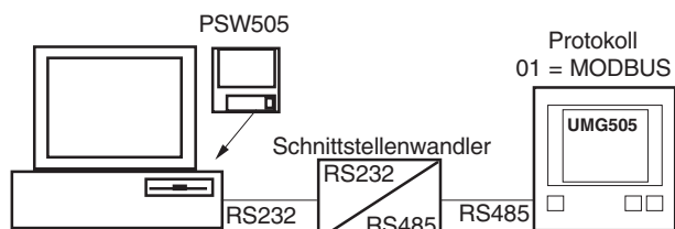
Abb. UMG505 mit RS485 Schnittstelle.
