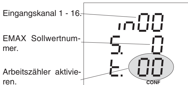
Abb. Arbeitszähler im UMG505.
