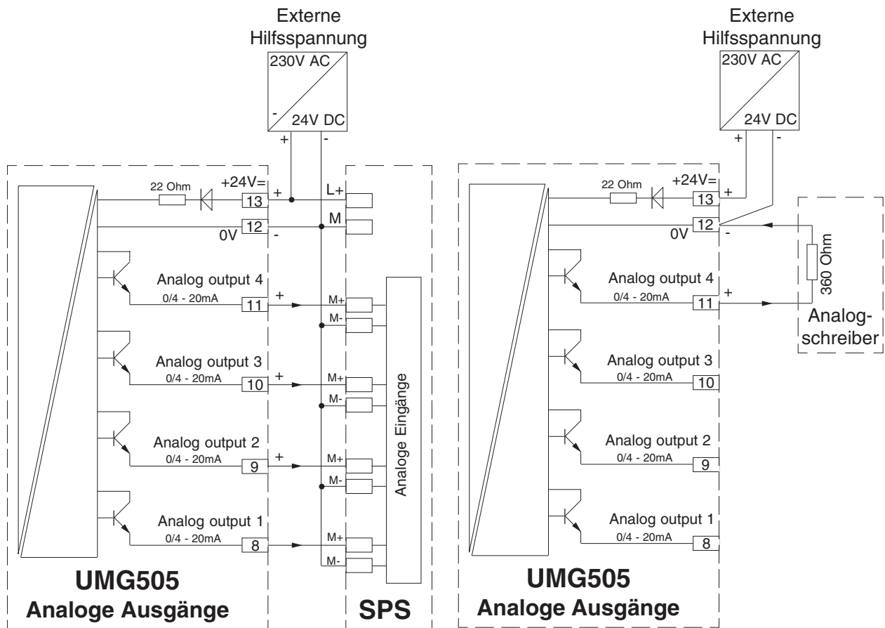
Abb. Anschluss eines Analogausganges an einen Analogschreiber.
