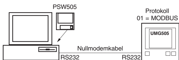
Abb. UMG505 mit RS232 Schnittstelle.
